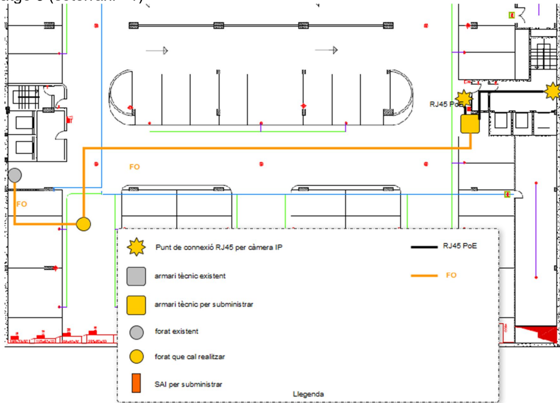
Imatge 3 (soterrani -1)
